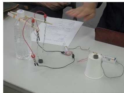
電磁誘導の実験装置 アルミブランコ(左)と クリップモーター(右)
